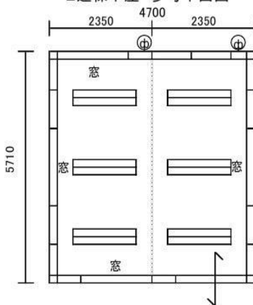
～2連棟平屋 参考平面図～
